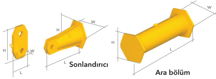
Bağlantı terminali
